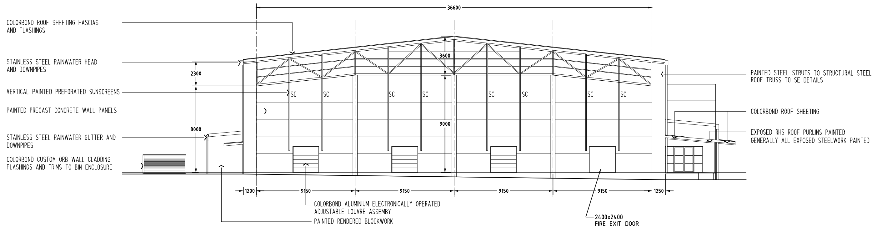
ELEVATION
